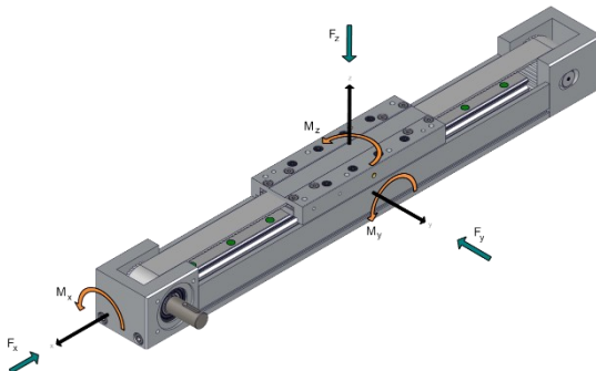
Abbildung 2: mechanische Belastungen
